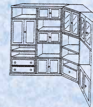
Art. 6564 Soggiorno componibile "Marte" Unit furniture L 270/180 H 234 P 60/35
