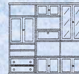
Art. 6562 Soggiorno componibile "Luna" Unit furniture L 270 H 234 P 60/35
